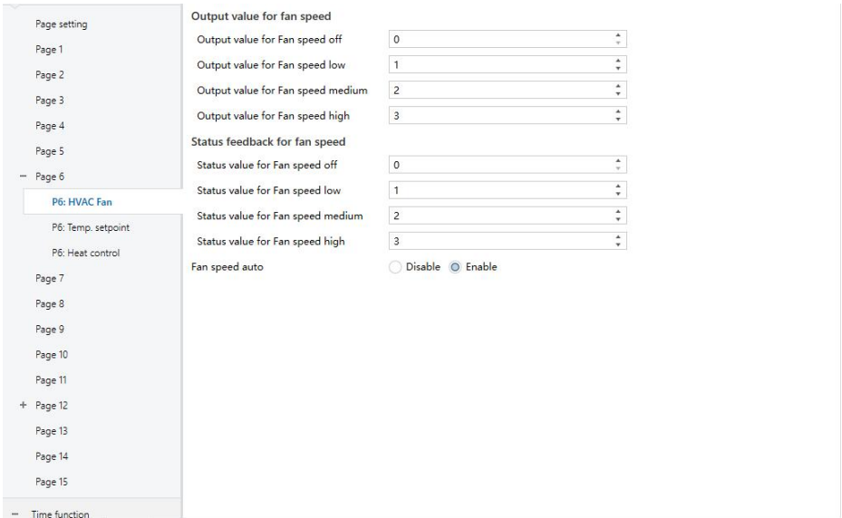
图 5.4.3 (2) “P x: HVAC Fan_1byte” 参数设置界面
