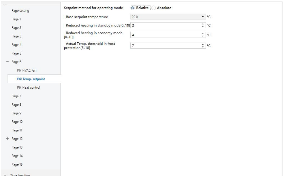
图 5.4.3 (3) “P x : Temp. Setpoint_Relative” 参数设置界面
