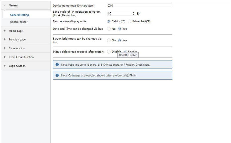
图 5.1_1 “General” 参数设置界面
