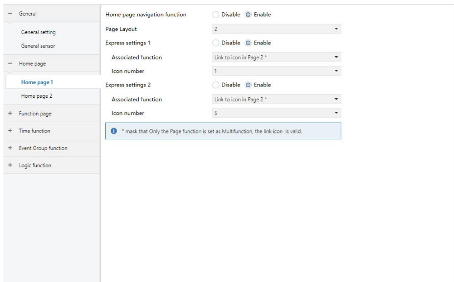
图 5.3.1 “Home Page x” 参数设置界面
