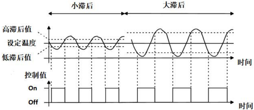
图 5.4.3 (6) 两点控制方式下滞后对控制值开关动作的影响 (加热)
